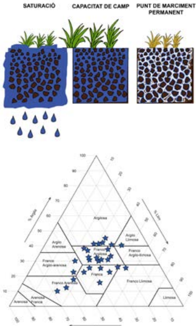
Fig. 41. Superior: La Capacitat de Retenció d'Aigua Disponible (CRAD) és la diferència entre la Capacitat de Camp (CC) i el Punt de Marciment Permanent (PMP9). Inferior: Triangle USDA de les textures del sòl.
